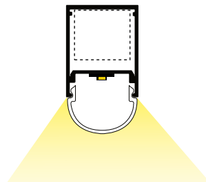
LN1-RL LINEA 1 ROUND LENS
