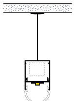
PENDANT MOUNT
