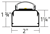
CV2
